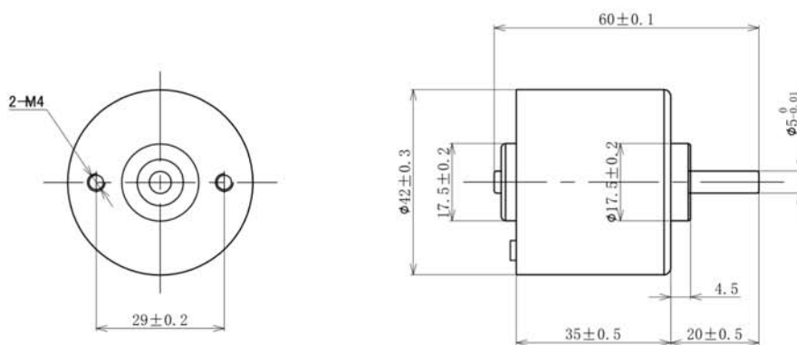
直流无刷电机 BLDC MOTOR
