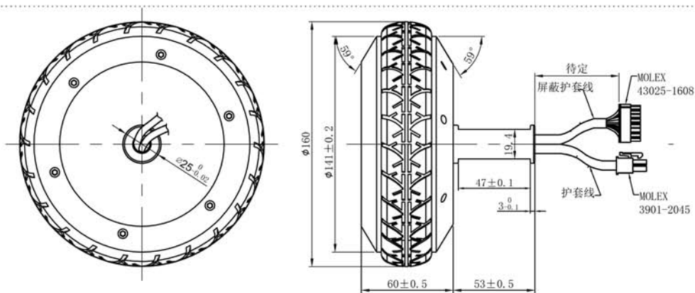
直流无刷电机 BLDC MOTOR
